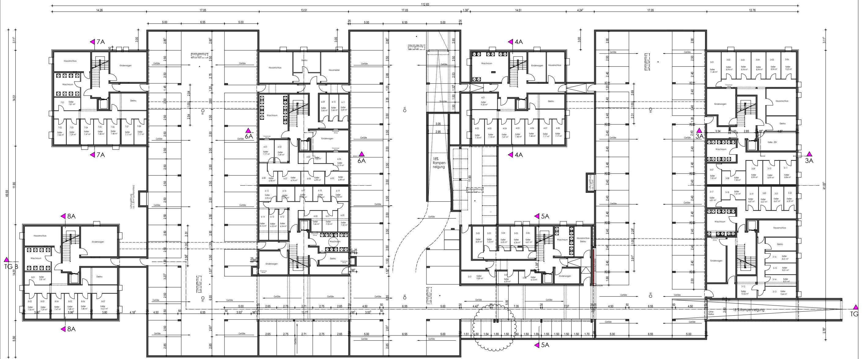
Grundriss Untergeschoss/ Tiefgarage Haus 3 bis 8
